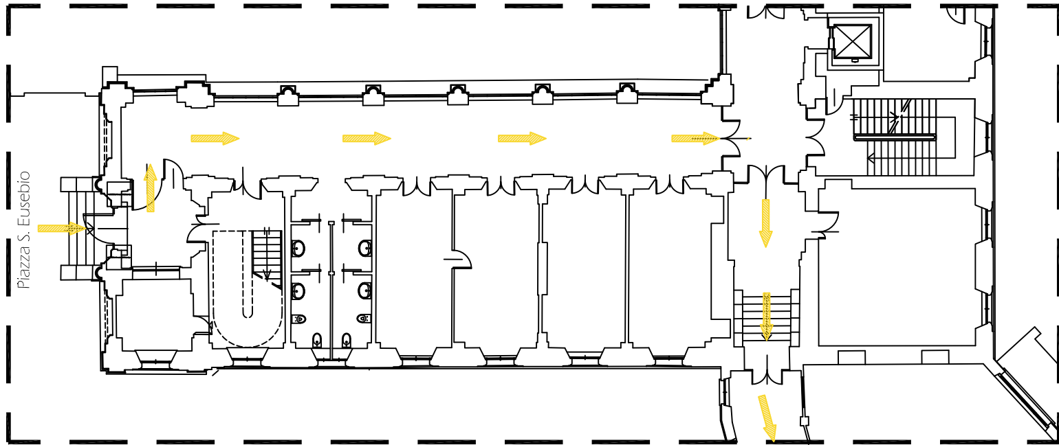
Piano Primo - Edificio A
